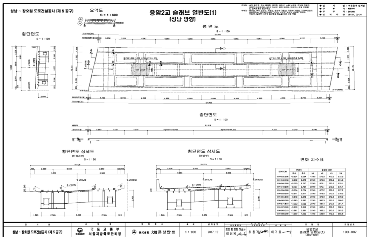
【그림 2.1.3】 응암2교(성남) 슬래브 일반도
