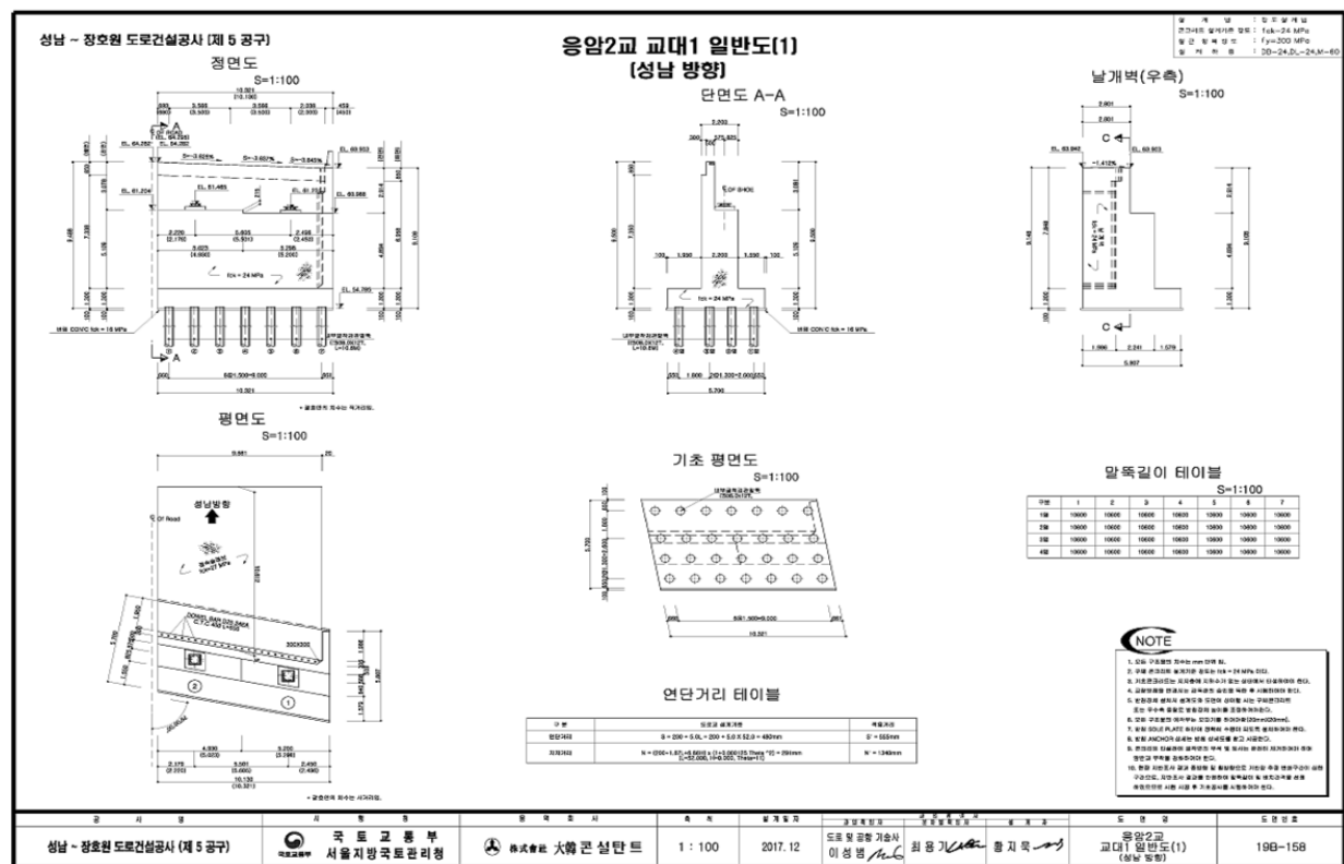
【그림 2.1.4】 응암2교(성남) 교대일반도(1)
