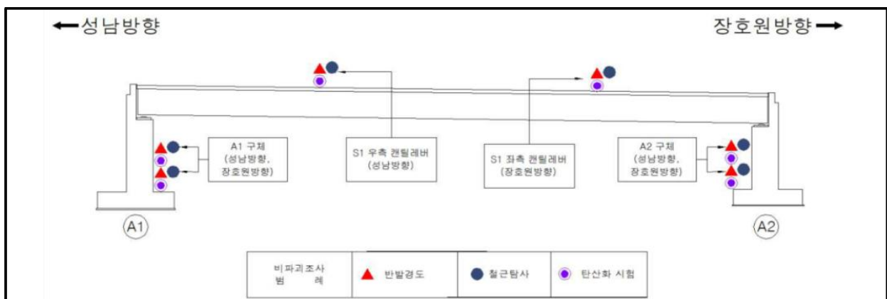
【그림 2.3.1】 콘크리트 내구성조사 위치도
