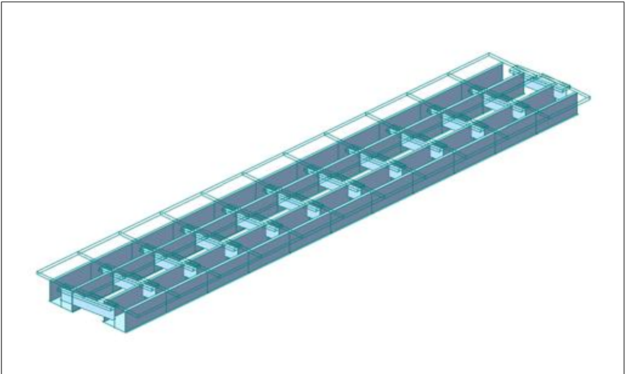
【그림 2.4.1】 응암2교(성남) 교량 구조해석 모델링
