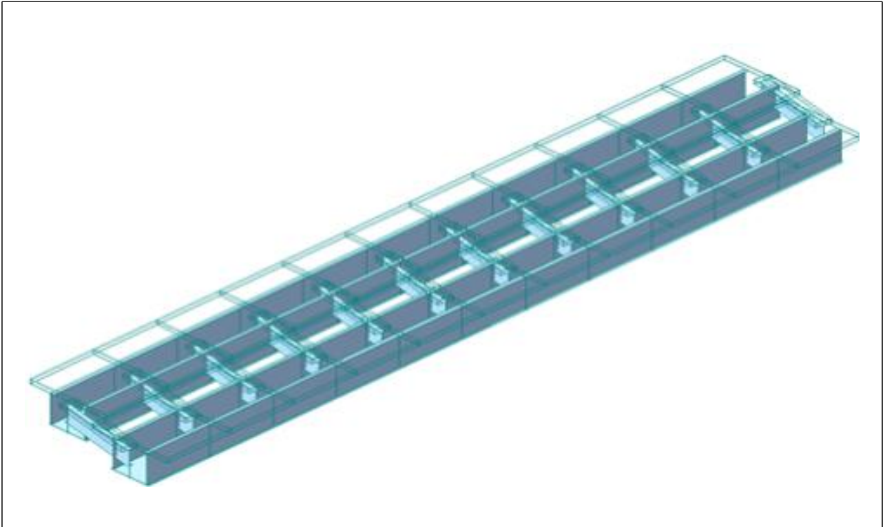
【그림 2.4.2】 응암2교(장호원) 교량 구조해석 모델링
